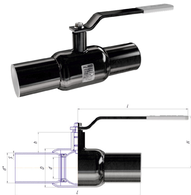
Габаритные и присоединительные размеры:
