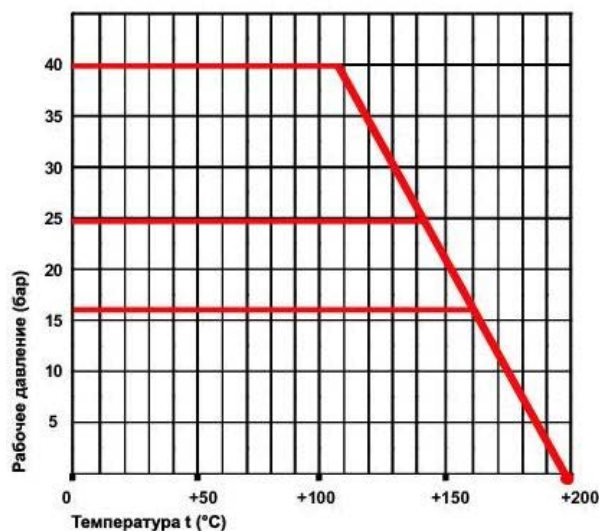
Зависимость "давление-температура" для седел из фторопласта-4
