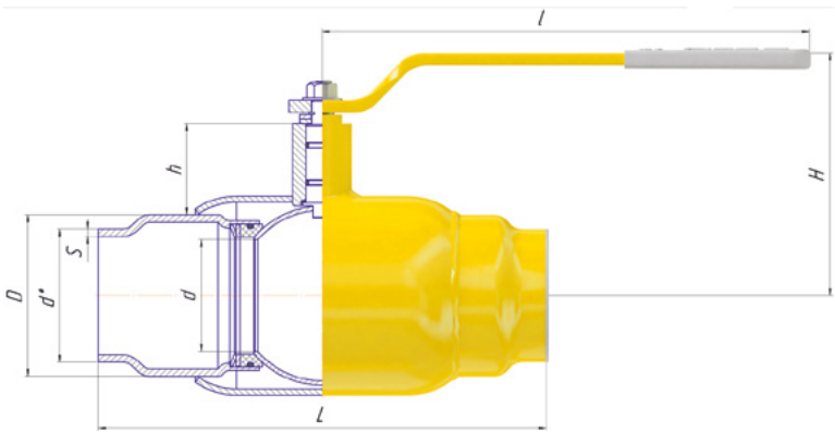
Габаритные и присоединительные размеры:
